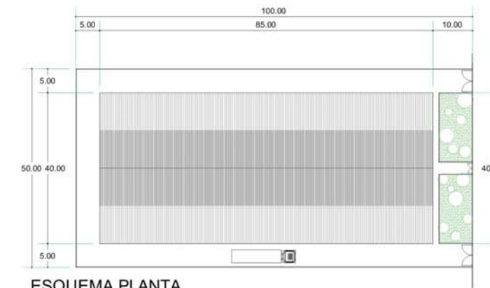
ESQUEMA PLANTA
